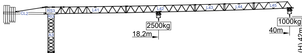
Cargas.Loads.Lasten.Charges.Cargas.Carichi.Yükler.ГРУЗОПОДЪЕМНОСТЬ
